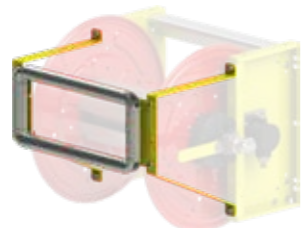
► SABIT OLARAK DUVARA KURULUMLAR İÇİN ÜST HORTUM KILAVUZU UPPER HOSE GUIDE FOR FIXED WALL INSTALLATION
