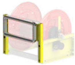
► SABIT OLARAK YERE KURULUMLAR İÇİN ÜST HORTUM KILAVUZU UPPER HOSE GUIDE FOR FIXED GROUND INSTALLATION
